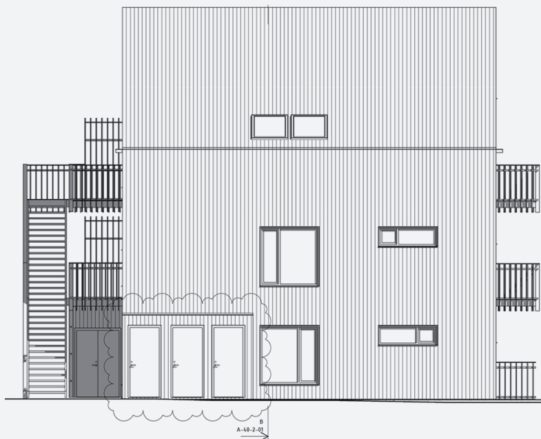
Fasad mot Öster
